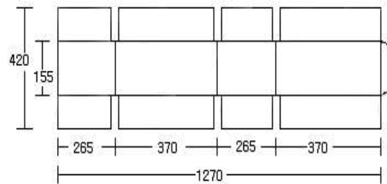
[그림9-6] 간미역 10kg 포장 설계도
