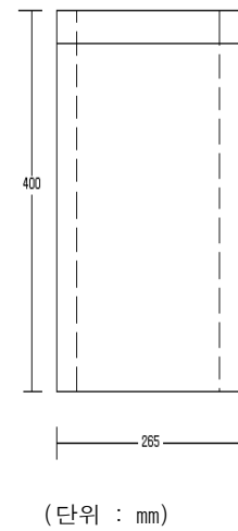
[그림2-4] 바지락 20kg 포장 설계도
