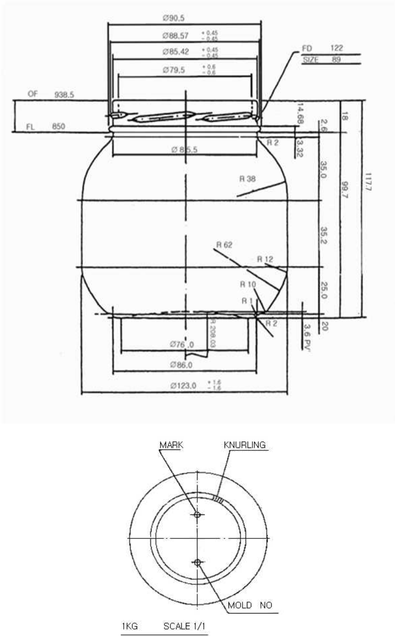
[그림7-1] 새우젓, 멸치젓 1kg 포장 설계도
