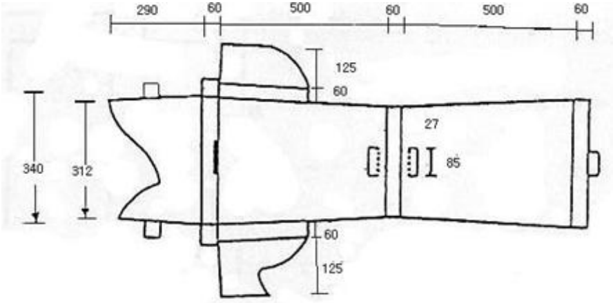
[그림4] 북어 10마리 포장 설계도
