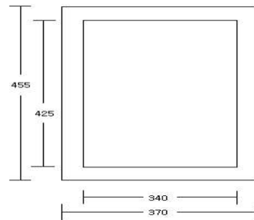
[그림9-4] 간미역 3kg 포장 설계도
