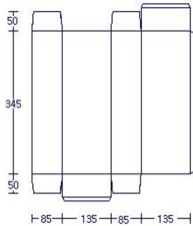
[그림8-1] 냉동오징어 2kg 포장 설계도
